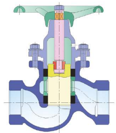
YPG 65-200
